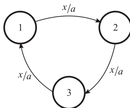
OBR. 17. Graf automatu z príkladu 3.13
