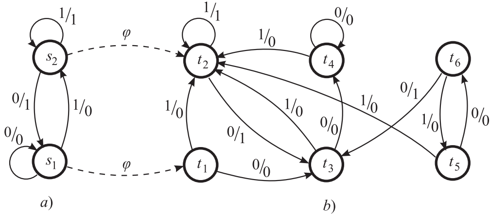
OBR. 39. Grafy automatov z príkladu 3.27
