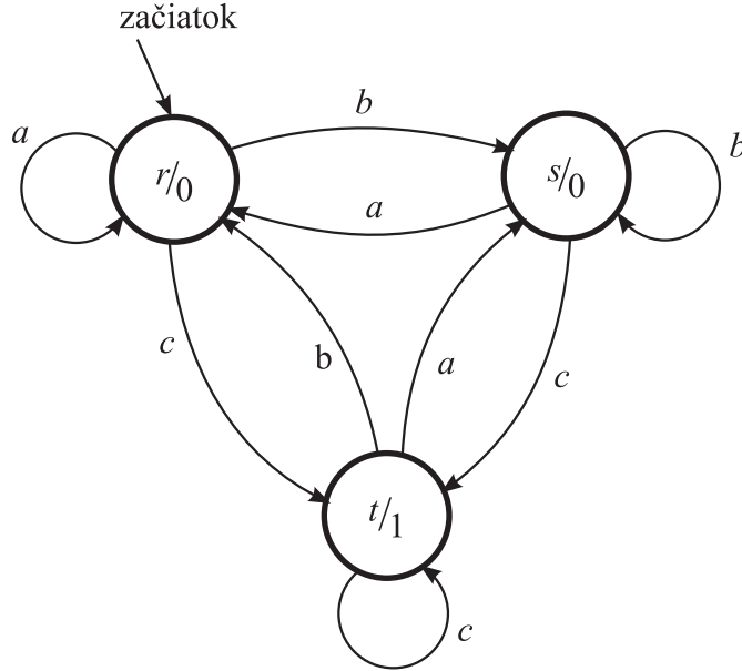
OBR. 13. Konečný akceptor z príkladu 3.8
