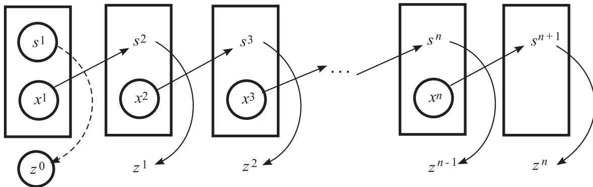
OBR. 9. Ilustrácia definície rozšírenej výstupnej funkcie Mooreovho automatu
