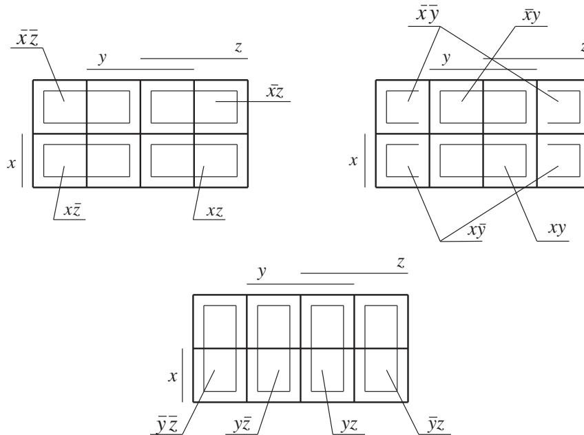
OBR. 48. Dvojice na Karnaughovej mape 3 premenných
