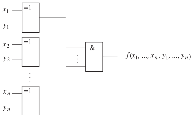
OBR. 24. Kombinačná logická sieť komparátora
