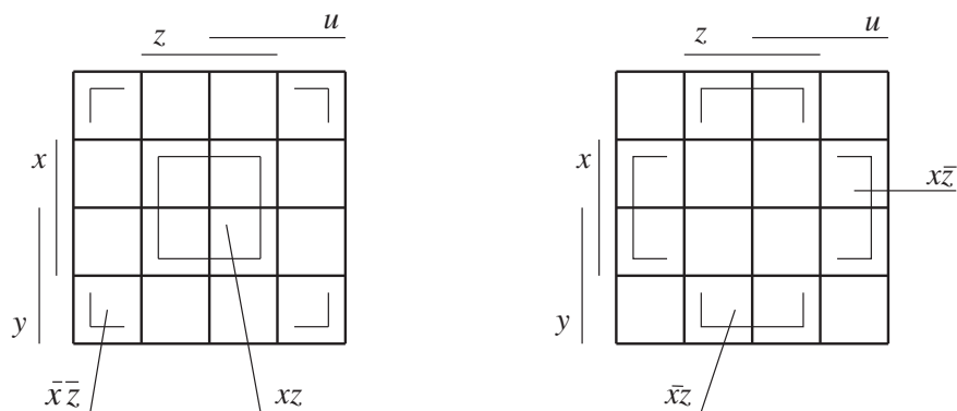
OBR. 51. Niektoré štvorice na Karnaughovej mape 4 premenných
