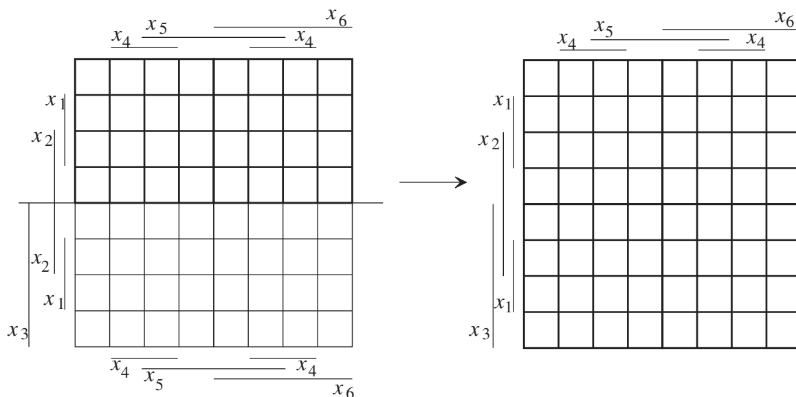
OBR. 42. Karnaughova mapa pre 6 premenných
