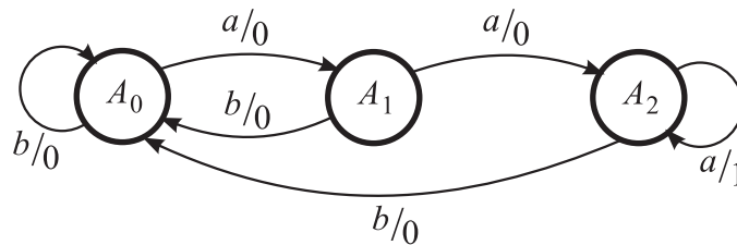
OBR. 32. Graf redukovaného automatu z príkladu 3.22
