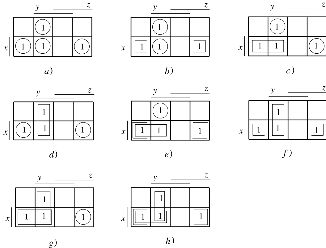
OBR. 57. NDF funkcie f z príkladu 2.44
