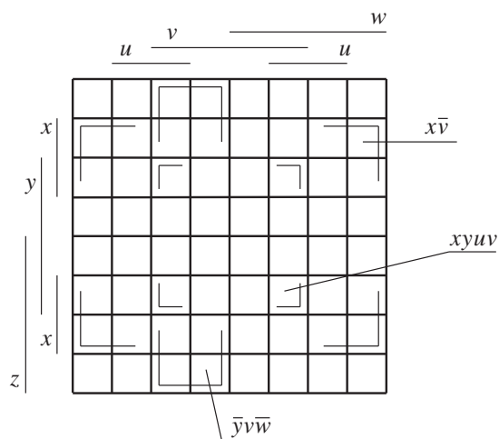
OBR. 54. Niektoré konfigurácie na Karnaughovej mape 6 premenných
