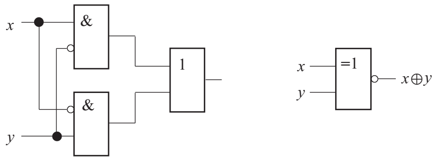
OBR. 19. Logický člen XOR
