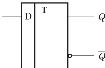
OBR. 14. D-preklápací obvod
