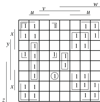
OBR. 56. NDF funkcie z príkladu 2.42
