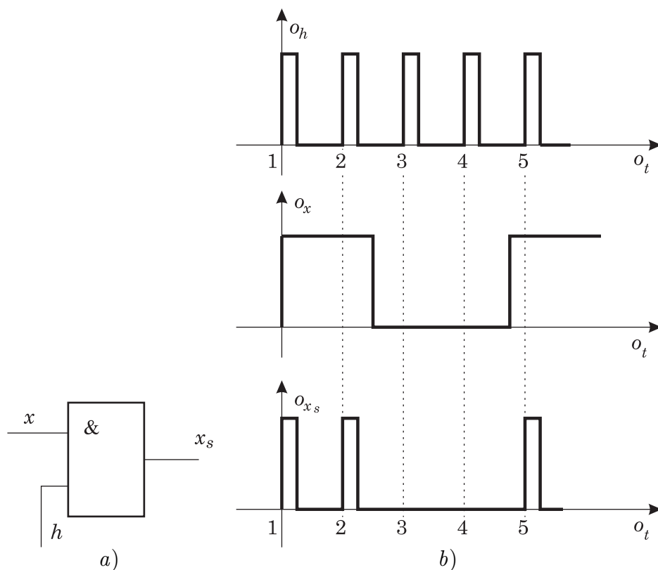
OBR. 29. Synchronizácia signálov
