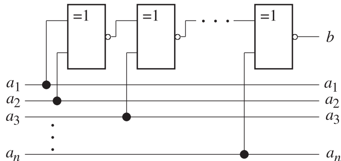
OBR. 26. Generovanie prídavného bitu na kontrolu parity
