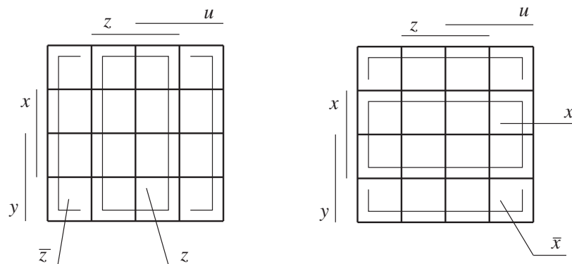
OBR. 52. Niektoré osmice na Karnaughovej mape 4 premenných
